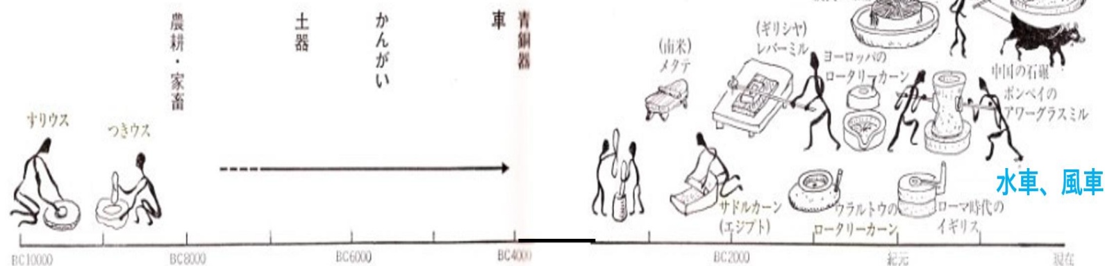
図1.2 白の1万年史年表
